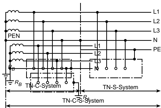
Abb. 13: a) TN-C-S-System
